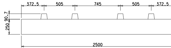
正面図
