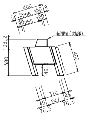
側面図
