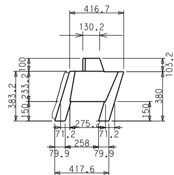
A-A断面図
