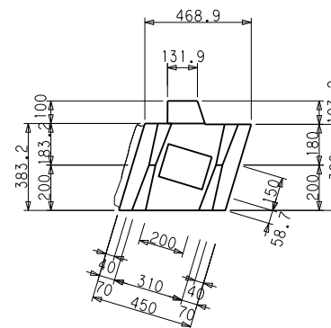
A-A断面図
