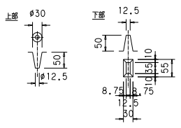
ガイドピン孔詳細 (S=1/10)
