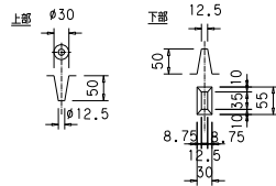
ガイドピン孔詳細 (S=1/10)
