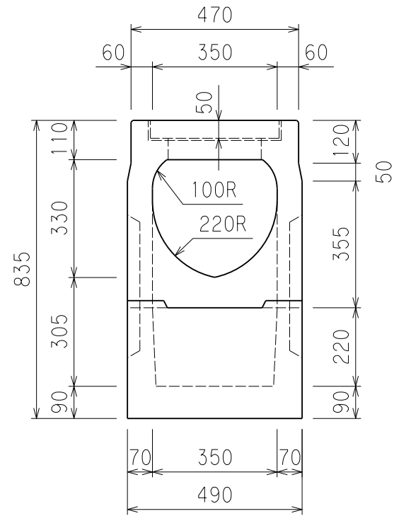
断面図
