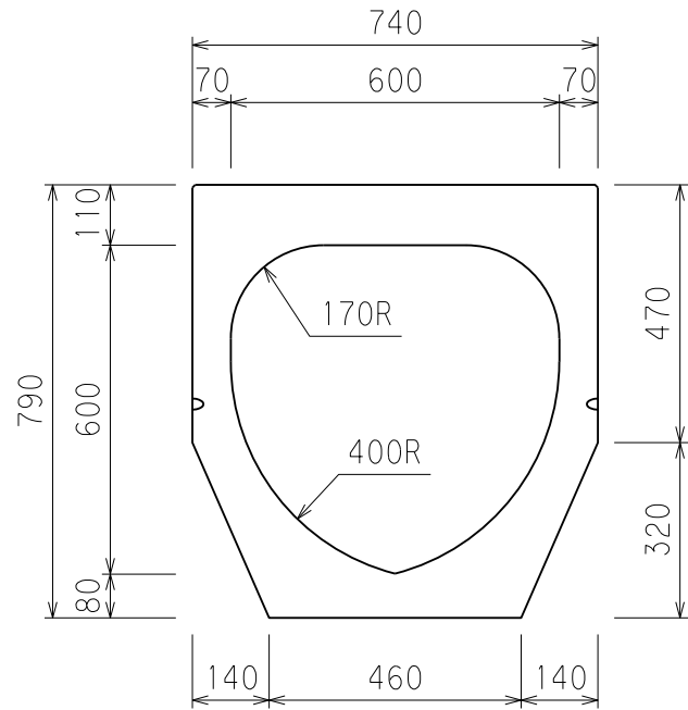
断面図
