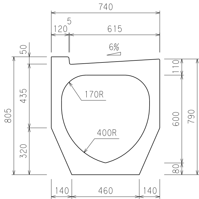
断面図
