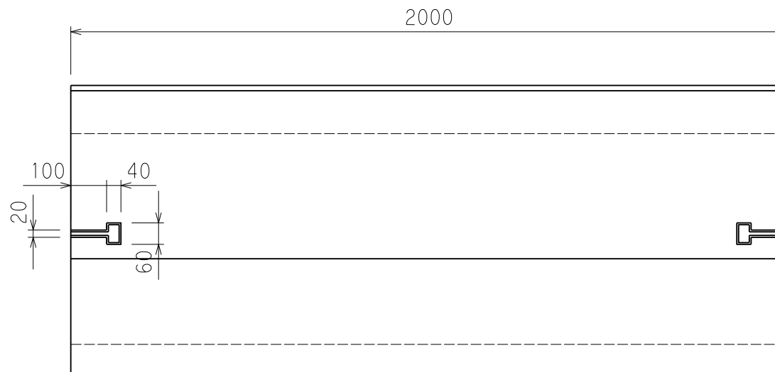
平面図
