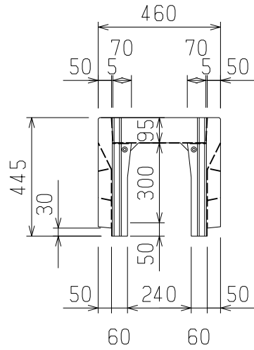
断面図
