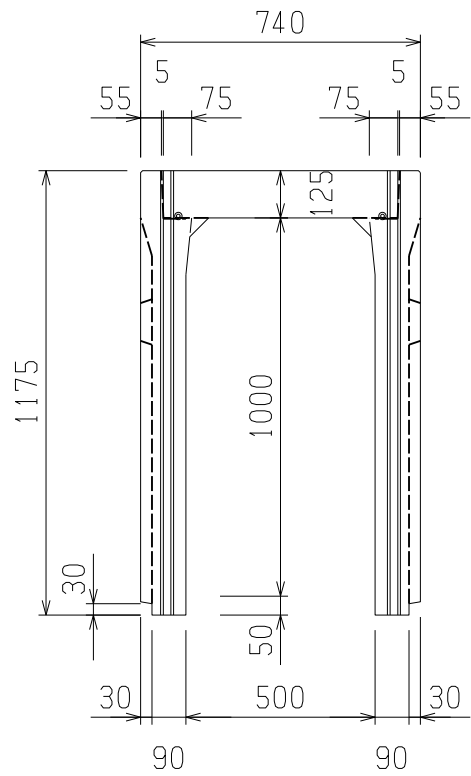
断面図
