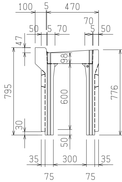
断面図
