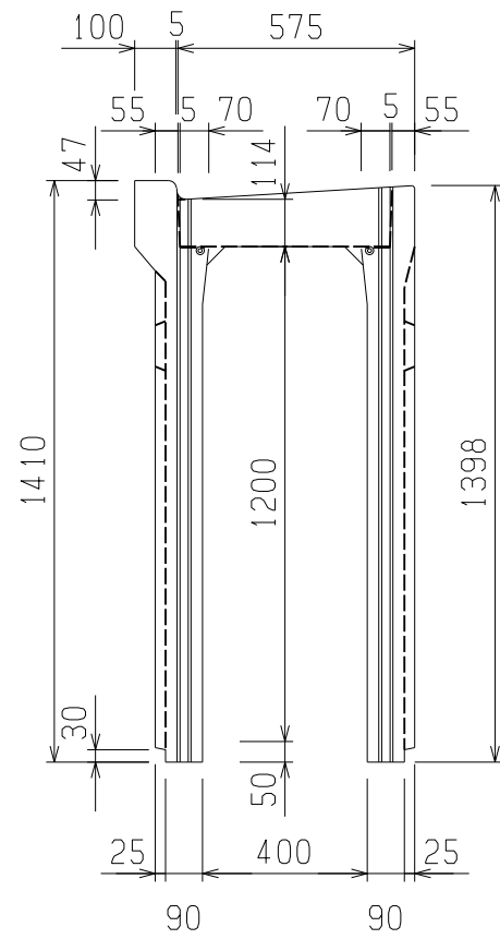
断面図
